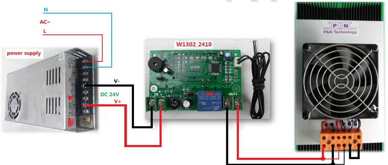
Original Terminal wiring scheme 橙色端子接线图
