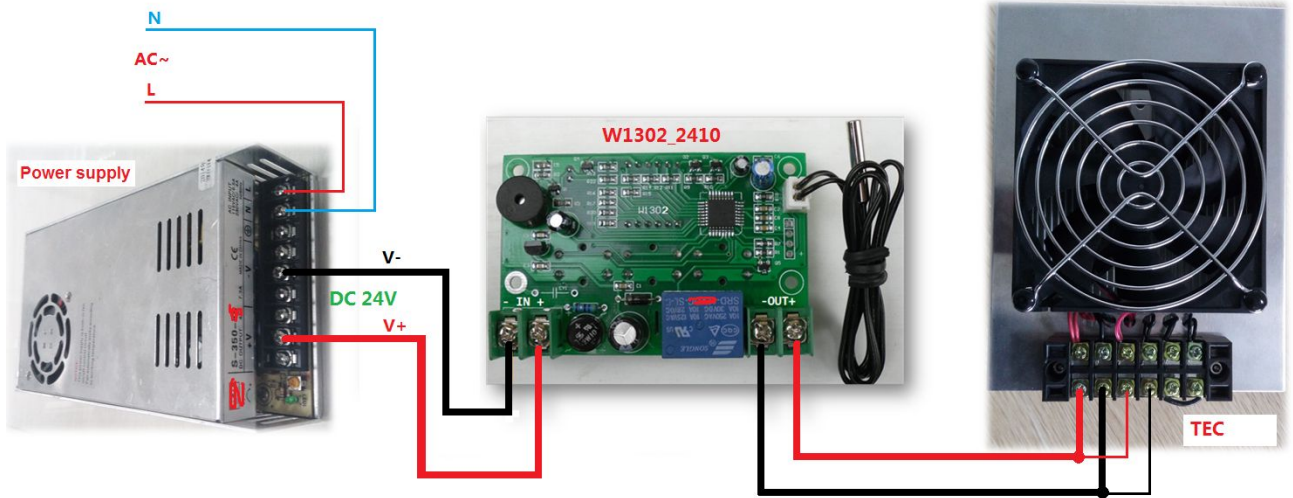
Original Terminal wiring scheme 橙色端子接线图
